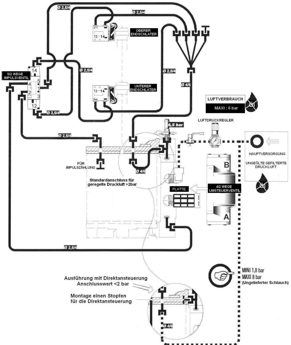
Pneumatik-Schema Luftmotor
